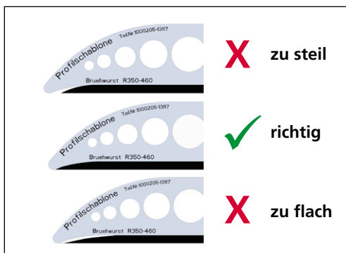
Bild 6-3 Messerprofil kontrollieren
