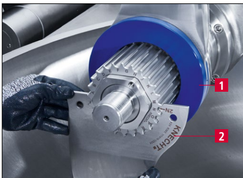
Bild 5-6 Füllstück (FST) einbauen
