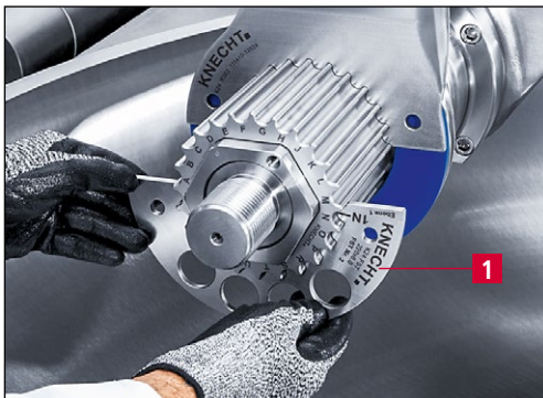
Bild 5-5 Auswuchtfüllstück (AWF) einbauen
