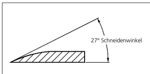
Bild 6-1 Schneidenwinkel
