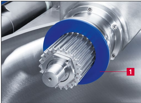
Bild 5-3 Zwischenring (ZR) einbauen
