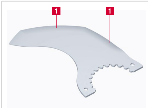
Bild 6-5 Schleifbereiche
