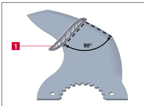
Bild 6-2 Profilschablone und ihre korrekte Position auf dem Messer
